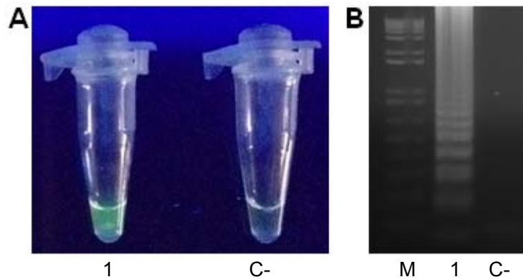
Figura 16: SYBR Green como método de visualização de resultados. Foram utilizados 1) 30 ng de DNA total de A. aegypti infectado por wMel . Após incubação, (A) 1 \mu l de SYBR foi adicionado em cada tubo e foram visualizados sob luz UV (302 nm). Para confirmação, (B) o produto de cada tubo foi aplicado em gel de agarose a 1,5% corado com brometo de etídeo. M: Marcador de peso molecular 1kb plus; C-: controle negativo.
