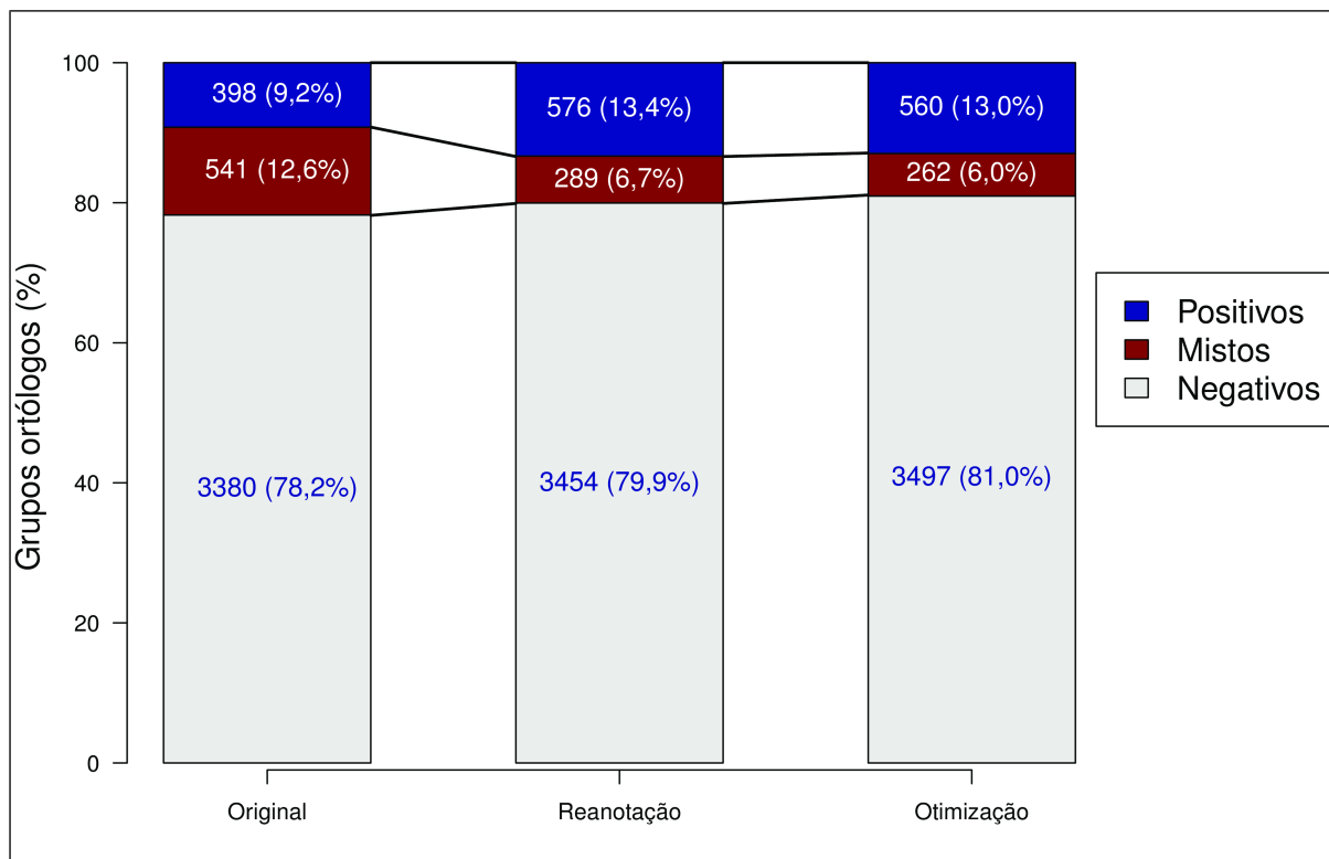
Figura 19: Reclassificação de grupos ortólogos após a otimização das configurações de predição de peptídeo sinal. Após a reanotação de proteínas, novos valores de corte para os parâmetros de predição foram selecionados e os resultados das predições foram usados na reclassificação de grupos. Os novos valores de corte para os parâmetros de predição foram: NN-Sum = 4; D-escore = 0,48; Probabilidade sinal por HMM = 0,9.
