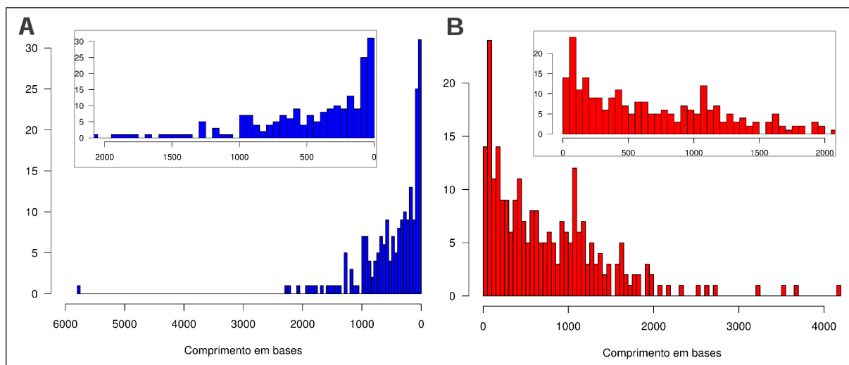
Figura 16: Distâncias entre a localização dos códons da metionina inicial do modelo gênico original e da metionina inicial proposta no novo modelo gênico. As reanotações resultaram no deslocamento da posição da metionina inicial para posições anteriores ( upstream ) (A) ou posteriores ( downstream ) (B) da metionina inicial original. Em detalhe um aumento na escala até 2.000 bases.
