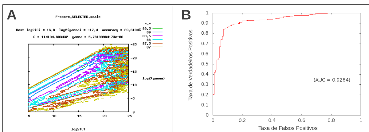
Figura 26: Treinamento do SVM. (A) Definição dos parâmetros C e \gamma . (B) Curva ROC calculada com os resultados de validação cruzada em 5 vezes e respectiva Área Sob a Curva (AUC).
