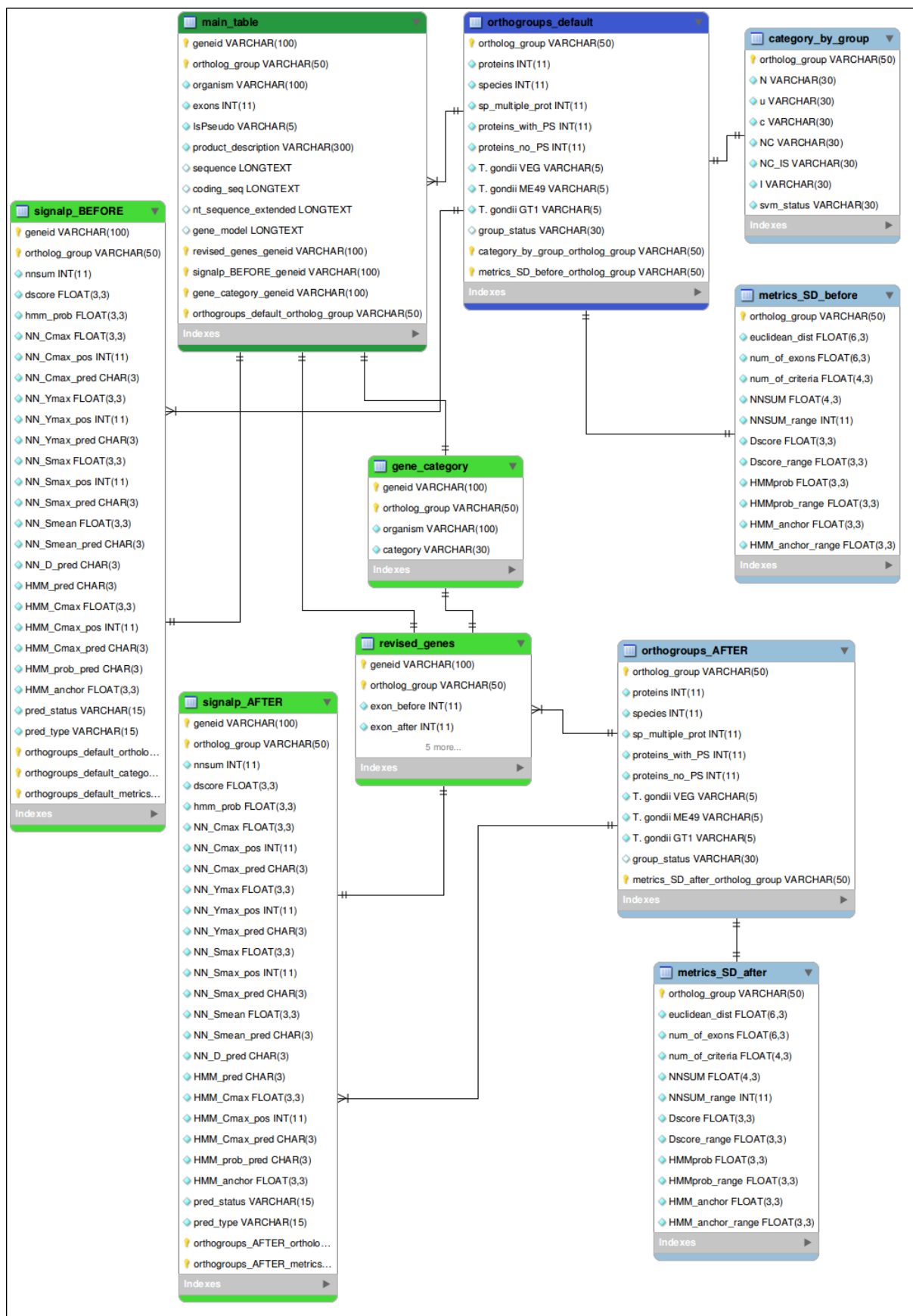
Figura 5: Diagrama da estrutura organizacional dos bancos de dados locais. As tabelas contendo informações sobre genes individuais estão destacadas em verde (em verde escuro a tabela com os dados retirados dos bancos do EuPathDB). As tabelas contendo informações sobre grupos de ortólogos estão destacadas em azul (em azul escuro a tabela resultante da classificação de grupos de ortólogos através das predições de peptídeo sinal, item 4.3). Destacadas em amarelo estão as
