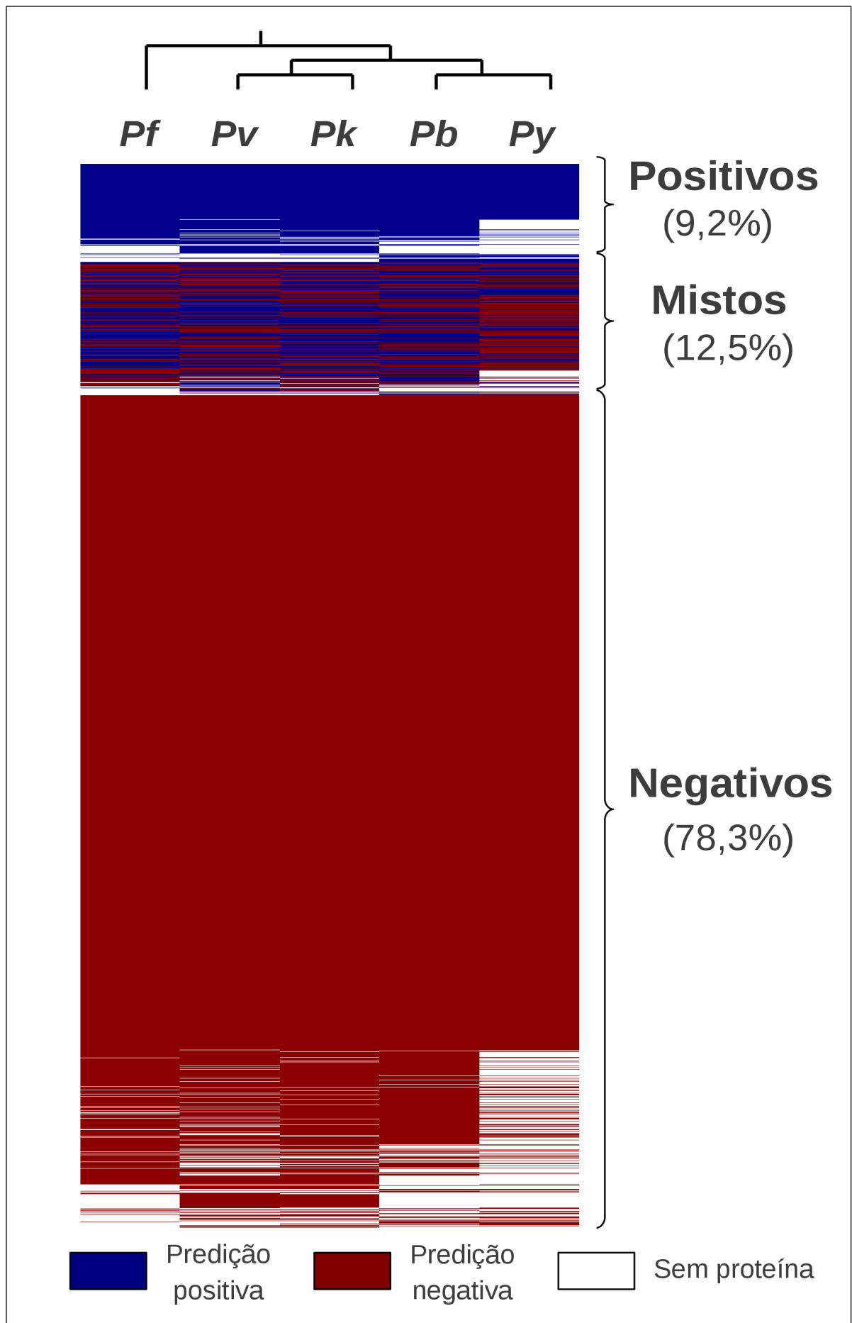
Figura 9: Distribuição dos grupos ortólogos classificados de acordo com a predição de peptídeo sinal de suas proteínas. Composição dos 4319 grupos por proteínas das diferentes
