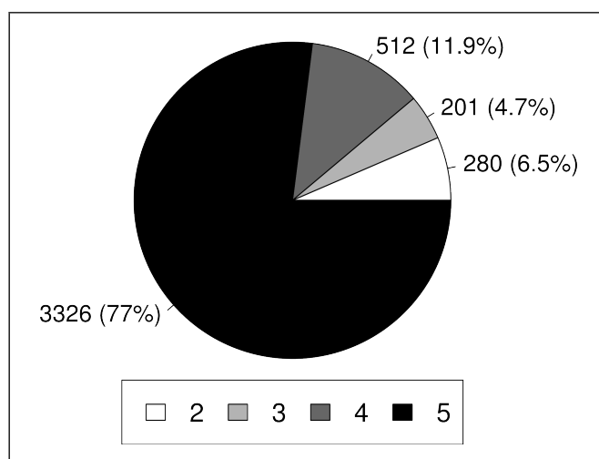
Figura 8: Total de proteínas compondo os grupos ortólogos. Os 4319 grupos ortólogos com no máximo uma proteína por espécie podem apresentar de duas a cinco proteínas. Foi feito o levantamento do número de proteínas em cada grupo.
